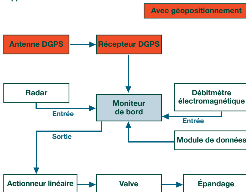
Figure 1 : Fonctionnement d'un système de dosage automatisé pour l'application de lisiers
